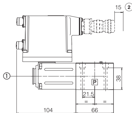
RZMO-AES-BP RZMO-AES-BC
